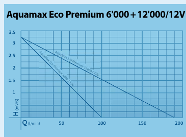
Pumpenkennlinie
