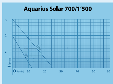
Pumpenkennlinie
