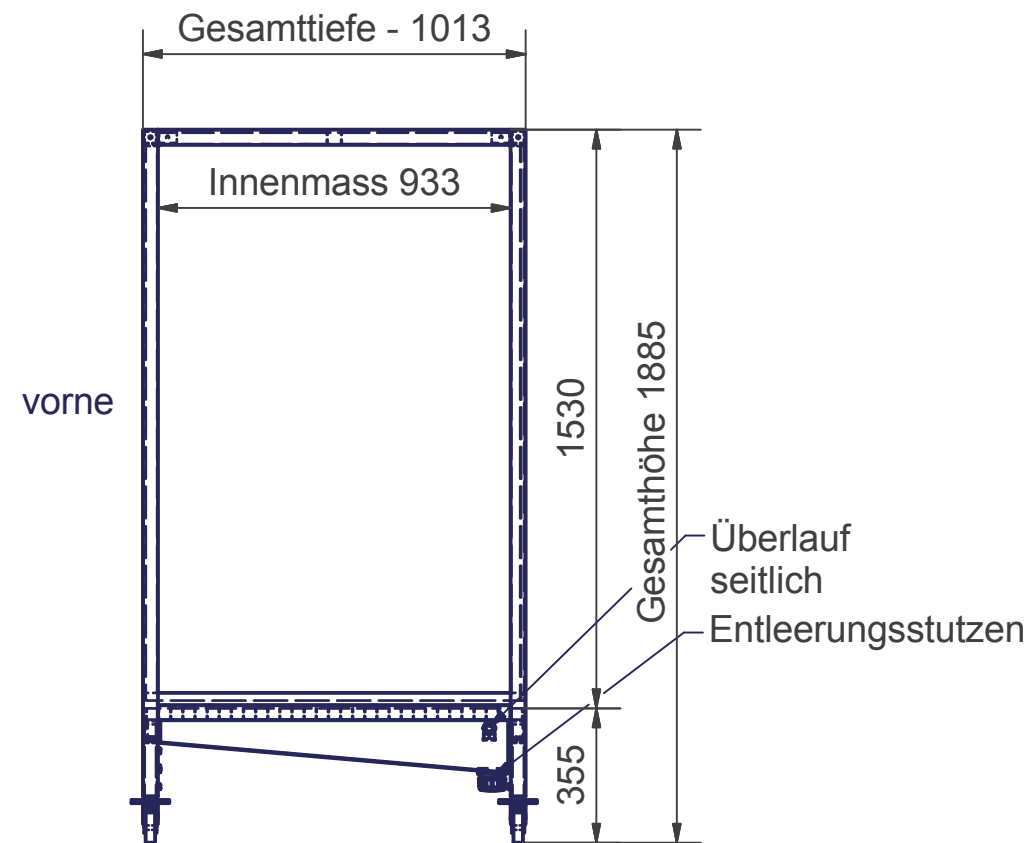
Seitenansicht ( 1 : 20 )
