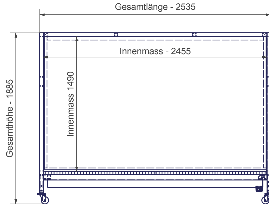
Ansicht ( 1 : 20 )
