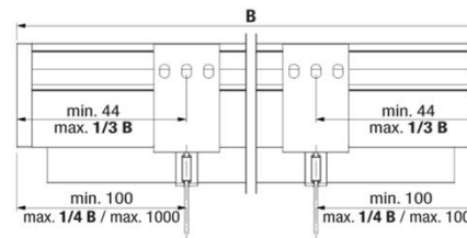
Drahtseilführung zweiseitig Eingerückt
