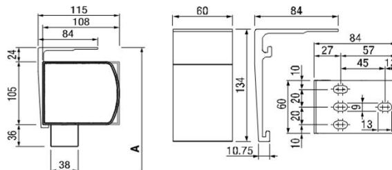
VA211-1 Deckenkonsole hoch
