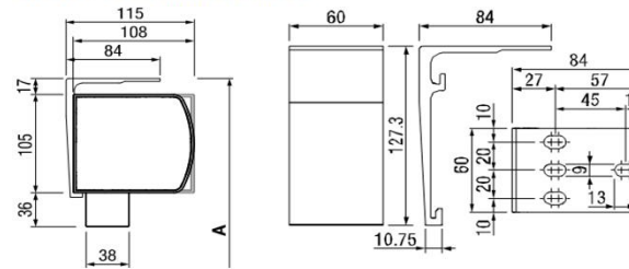
VA210-1 Deckenkonsole flach
