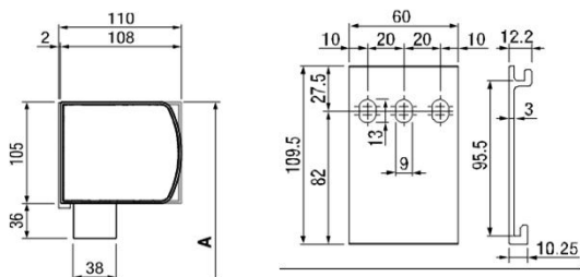
VA221-1 Wandkonsole
