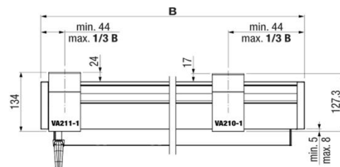
Verschiebbereich Deckenkonsole VA211-1 / VA210-1
