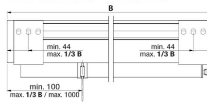
Drahtseilführung einseitig Eingerückt
