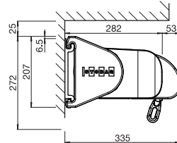
Wandmontage mit Volant-Plus Montage en façade avec Volant-Plus
