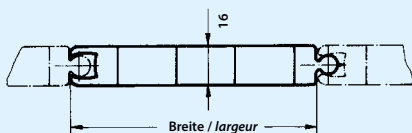
PVC-Doppelwandelemente Nut + Kamm 200/16, transparent Eléments à double parois en PVC 200/16, transparent, avec rainure et crête
