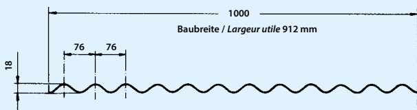
Polyesterplatten 76/18 Plaques en polyester 76/18 375 g
