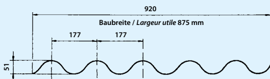
Polyesterplatten Eternitwellung 177/51 Plaques en polyester Ondulation Eternit 177/51 600 g
