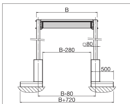
Mit Betonsockel
