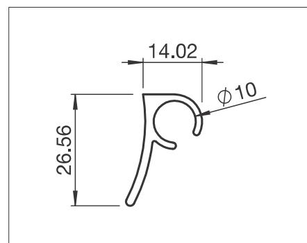
S551 Volantprofil
