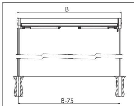
Version OS416/2 mit Bodenhülse
