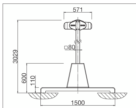
Mit Betonsockel
