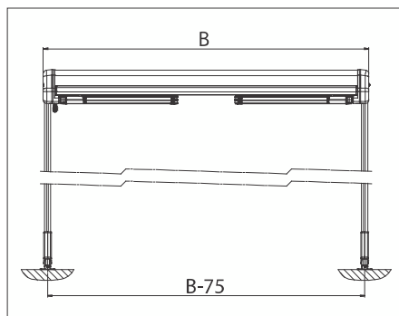
Version OS416/1 mit Querfuss
