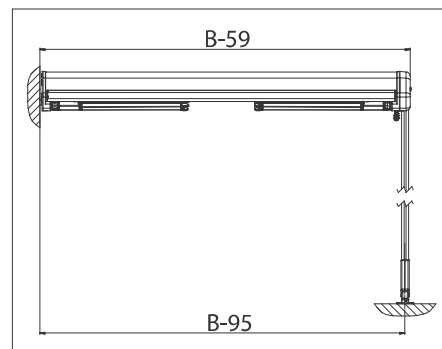
Version OS416/1 mit Querfuss und Wandhaltergarnitur OS4010/1
