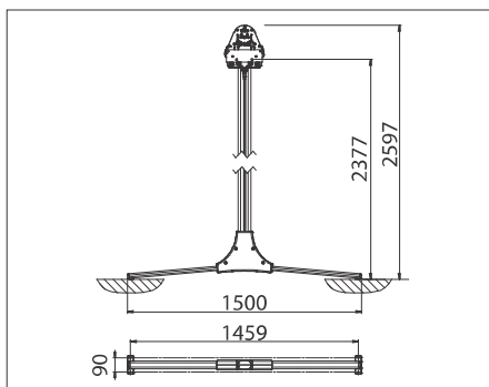
2-Beinversion OS416/1 mit Querfuss OS412
