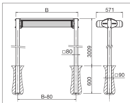
Mit Bodenhülsen
