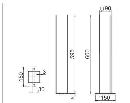
OS615 Bodenhülse
