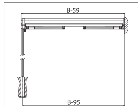
Version OS416/2 mit Bodenhülse und Wandhaltergarnitur OS4010/1
