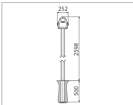
2-Beinversion OS416/2 mit Bodenhülse OS315
