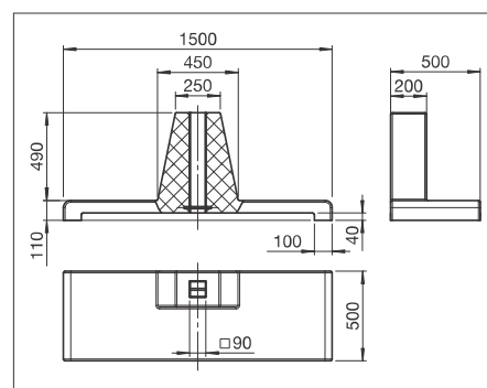
OS617 Betonsockel (ca. 186 kg)
